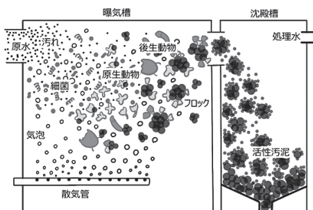
汚水処理の仕組み(株式会社 市川建設HPより抜粋) 活性汚泥の一部は肥料としてリサイクルしています。
